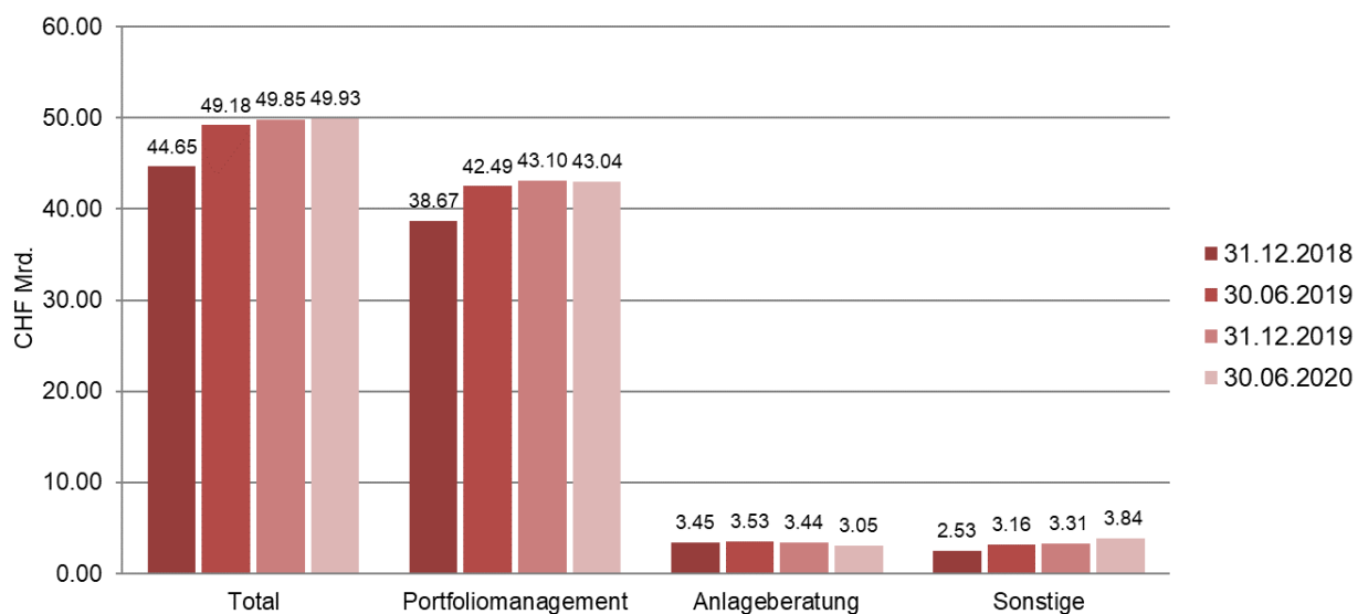
Abbildung 1: Entwicklung der Assets under Management nach Kategorien
